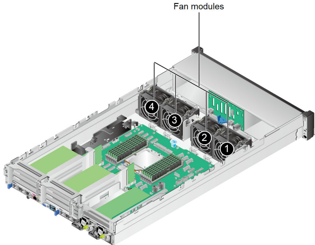
Figure 5-81 Positions of fan modules (example: 8038 fan module)
