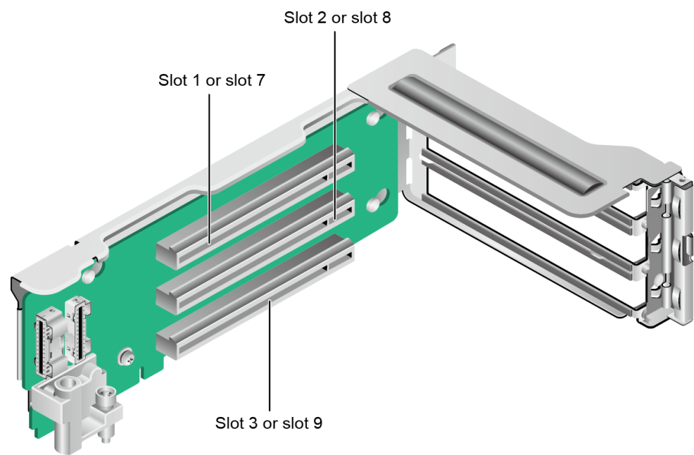
Figure 5-30 I/O module 1 or IO module 2
