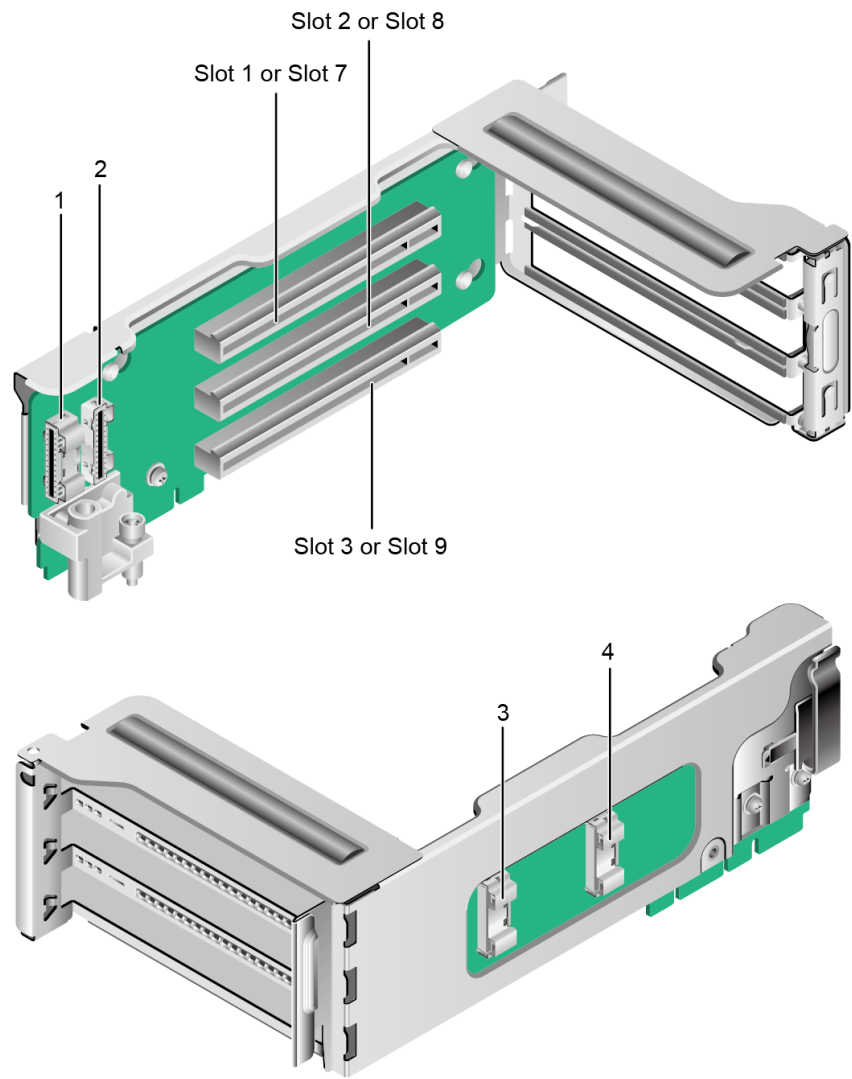
图 5-52 PCIe Riser 卡 1
