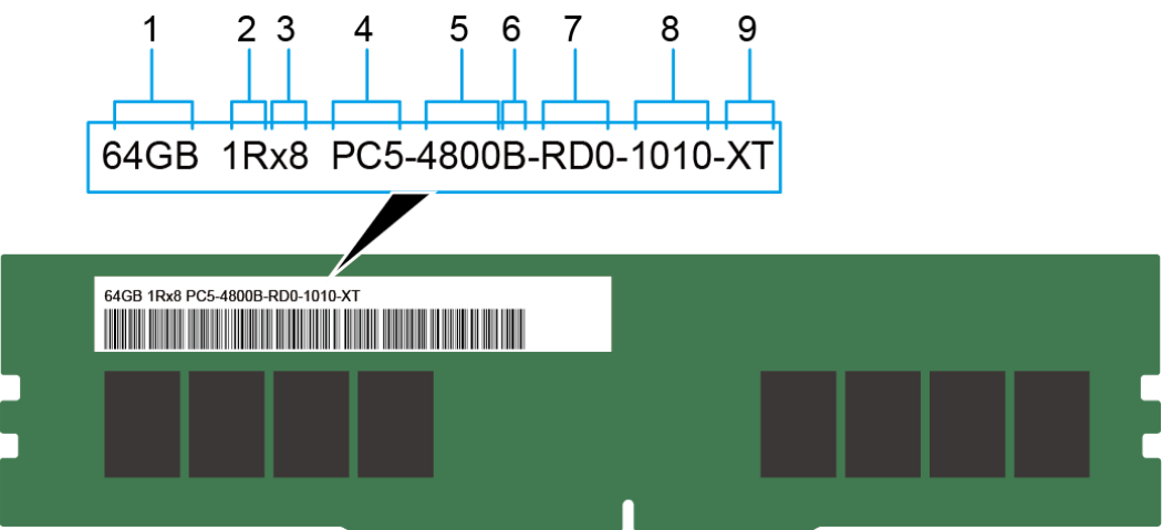
图 5-29 内存标识
