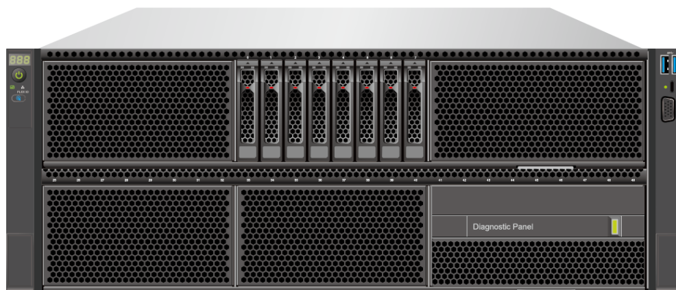
图 1-1 5885H V7 ( 示例：8x2.5 英寸硬盘配置 )
