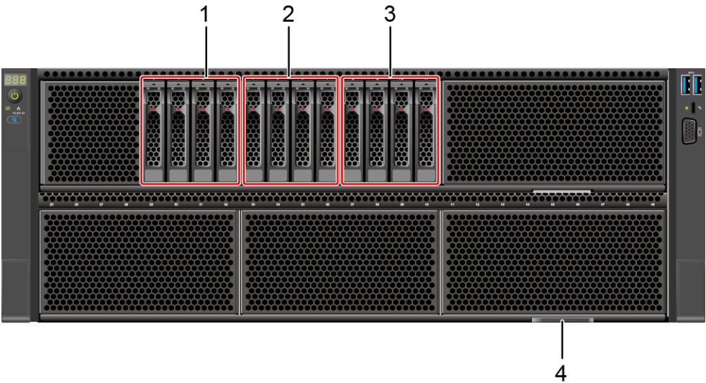
图 5-2 前面板外观
