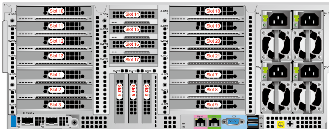
图 5-51 PCIe 插槽
