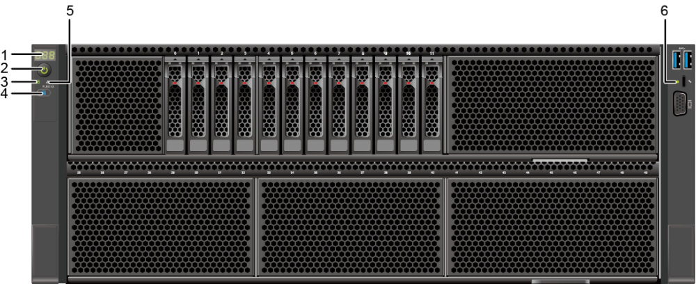
图 5-9 前面板指示灯和按钮
