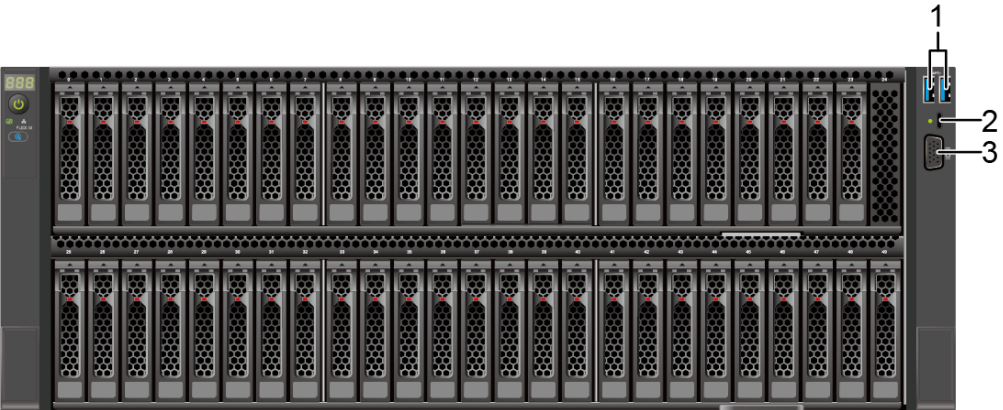
图 5-21 前面板接口
