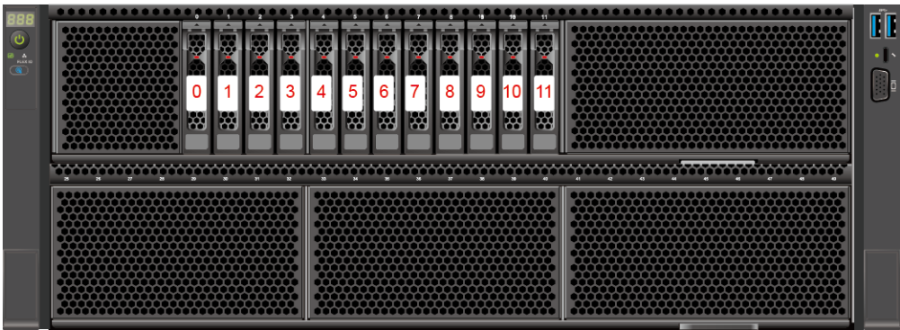
图 5-37 硬盘编号
