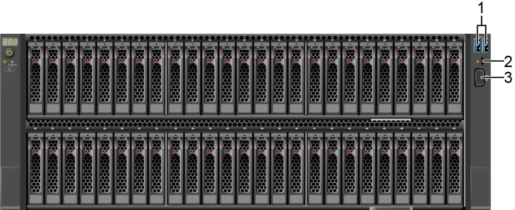
图 5-20 前面板接口
